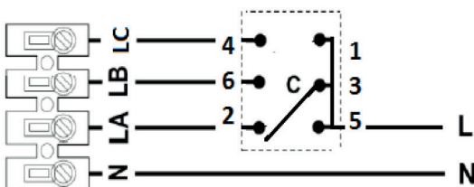
schéma zapojení COM 3 s TD MIXVENT 3V a TH MIXVENT 3 V
