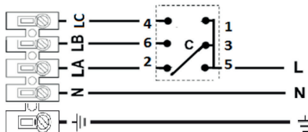
schéma zapojení COM 3 s TD MIXVENT 3V a TH MIXVENT 3 V se zemnicím vodičem
